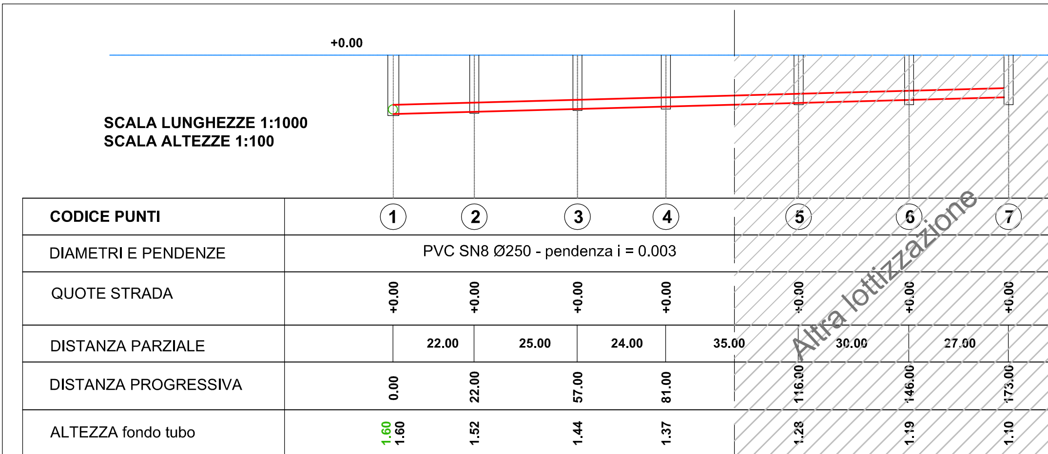
Profilo longitudinale predisposizione acque nere
